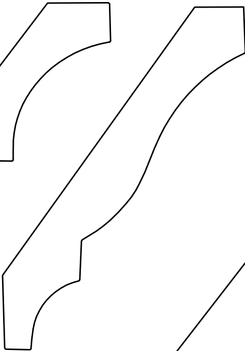
MV346 - 11/16" x 4 1/4"
